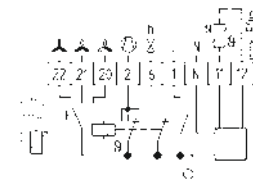
KLR-E 525 52 hp
